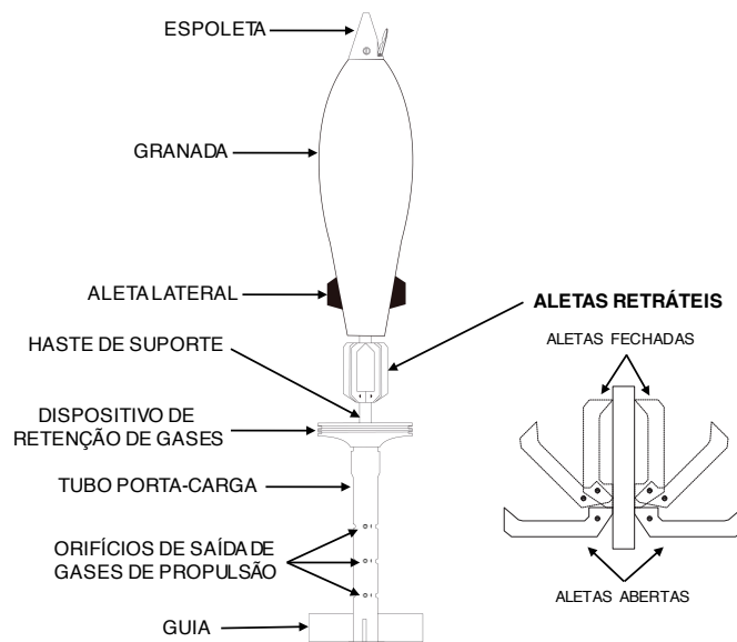
Figura 38 – Vista externa do conceito de munição de morteiro. Fonte: Autor.
