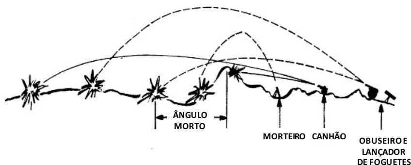
Figura 10 – Esquema de trajetórias de sistemas balísticos. Fonte: Adaptado de Guia de Operações Militares (2012).
