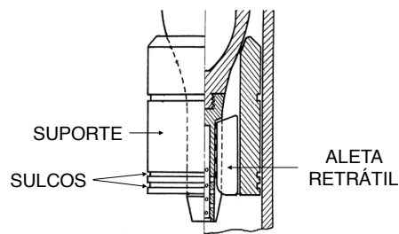
Figura 21 – Esquema de solução conforme o requisito técnico RT16. Fonte: Adaptado de Hans (1955).
