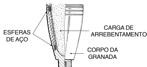
Figura 30 – Esquema de solução conforme o requisito técnico RT27. Fonte: Adaptado de Diehl GMBH & CO (2008).
