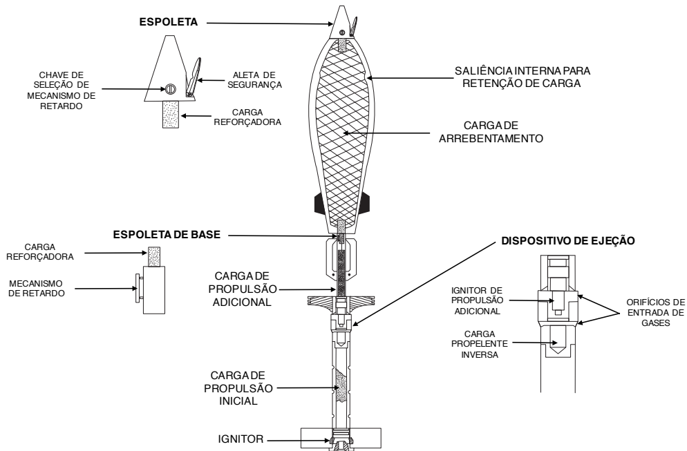
Figura 37 – Vista interna do conceito de munição de morteiro. Fonte: Autor.
