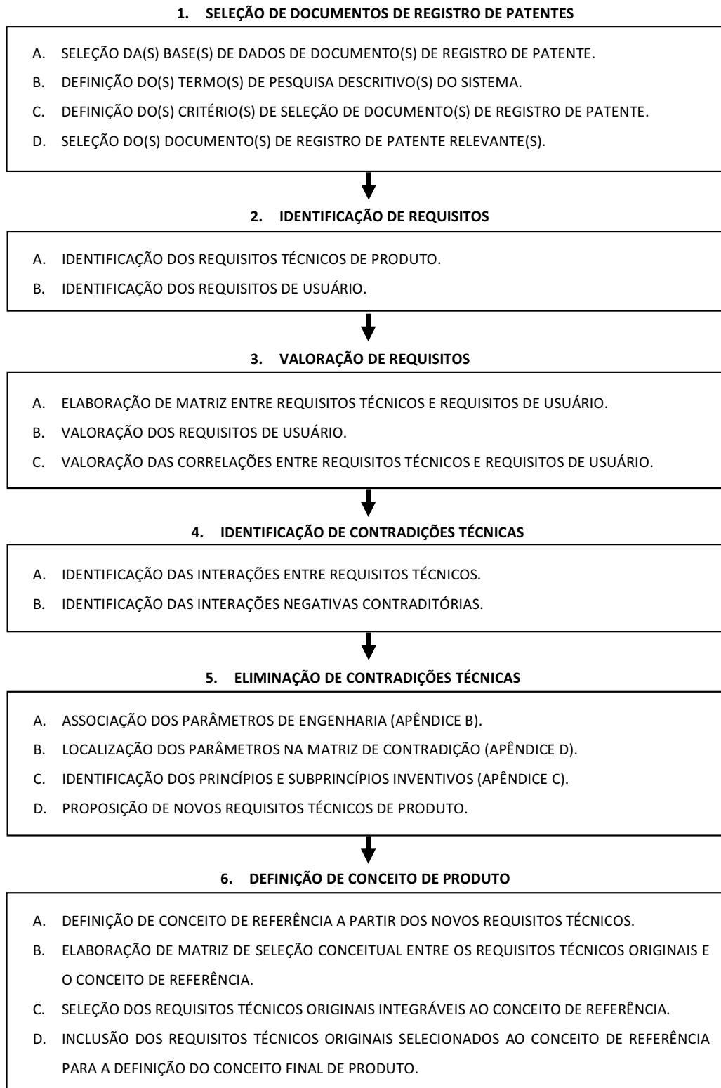
Figura 9 – Protocolo de Otimização Sistemática de Requisitos de Engenharia. Fonte: Autor.
